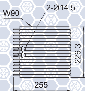
F2-00759 COROLLA / SERA
