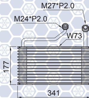
F8-00774 SUNFIRE / CAVALIER
